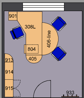
Půdorys varianta 5
