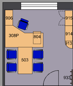
Půdorys varianta 8
