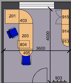
Půdorys varianta 1
